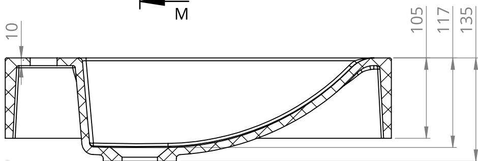
PRZEKRÓJ N-N
