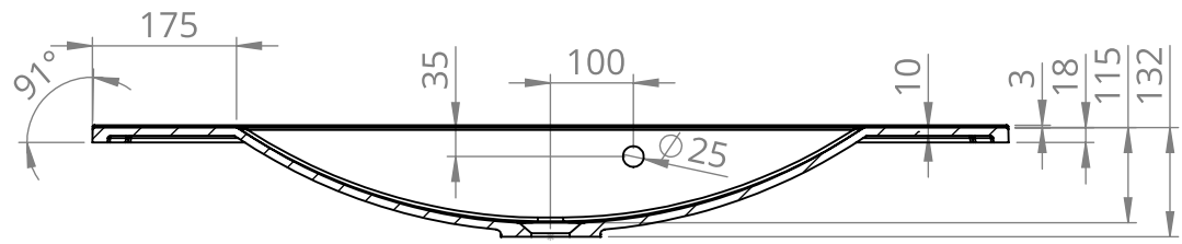
PRZEKRÓJ M-M
