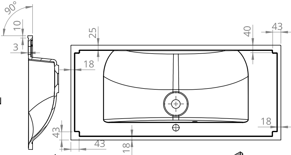
PRZEKRÓJ M-M
