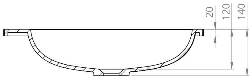
PRZEKRÓJ N-N SKALA 1 : 7
