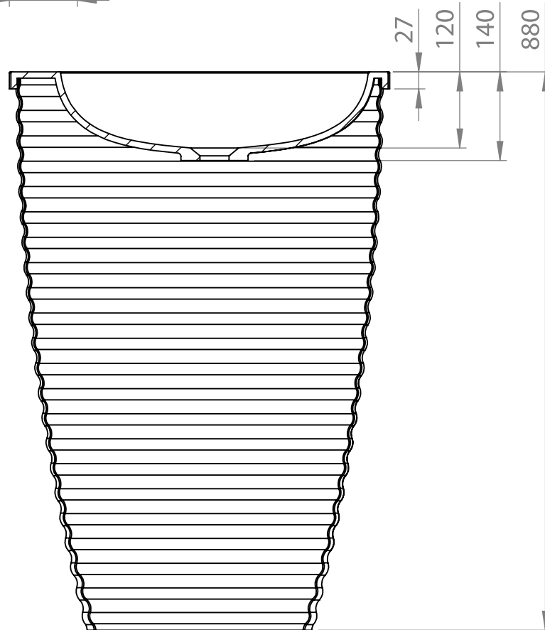
PRZEKRÓJ N-N SKALA 1 : 10
