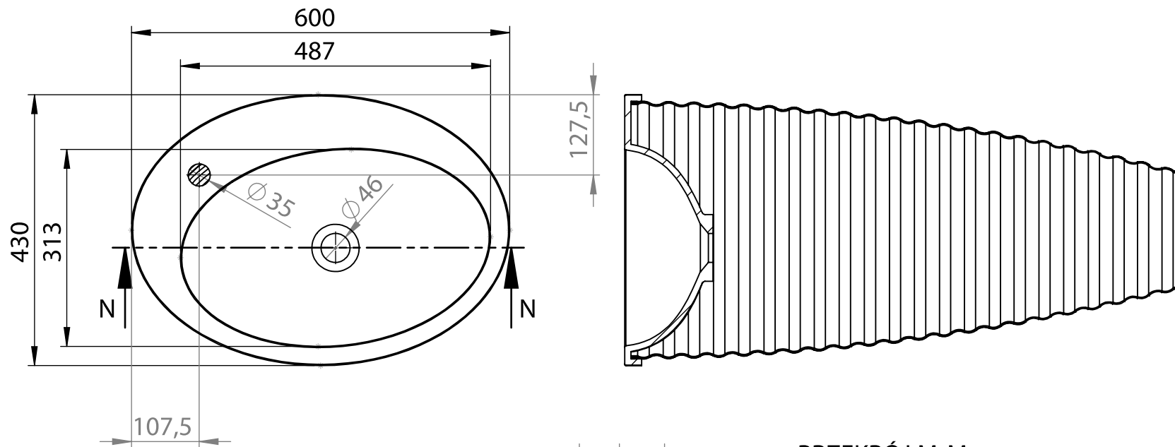
PRZEKRÓJ M-M SKALA 1 : 10
