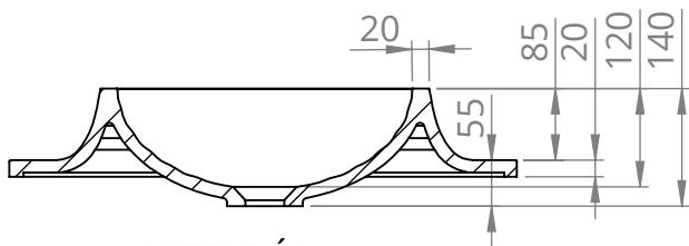
PRZEKRÓJ O-O SKALA 1 : 10
