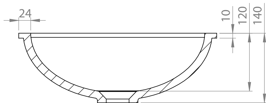
PRZEKRÓJ M-M SKALA 1 : 6
