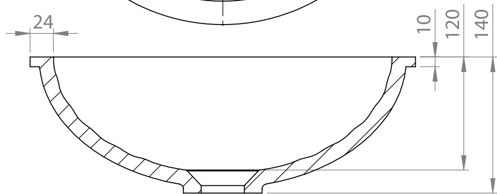
PRZEKRÓJ N-N
