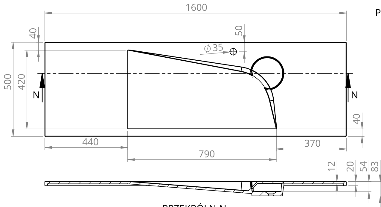
PRZEKRÓJ N-N SKALA 1 : 12
