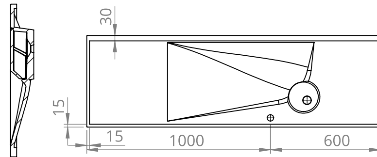
PRZEKRÓJ M-M SKALA 1 : 12
