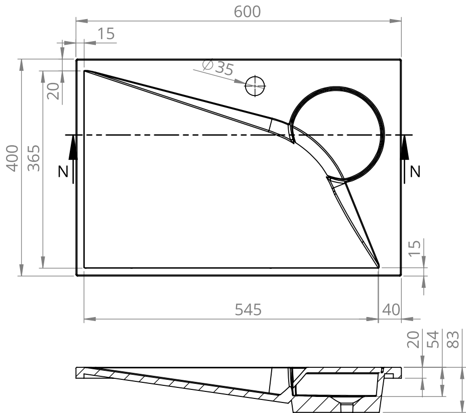
PRZEKRÓJ N-N SKALA 1 : 7
