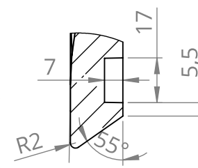
PRZEKRÓJ N-N SKALA 1 : 10
