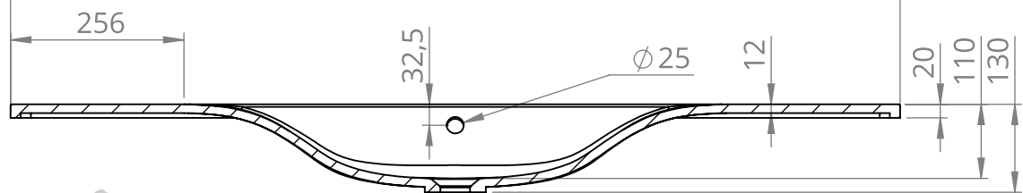
PRZEKRÓJ M-M SKALA 1 : 10
