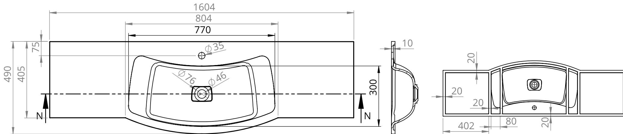
PRZEKRÓJ M-M SKALA 1 : 12
