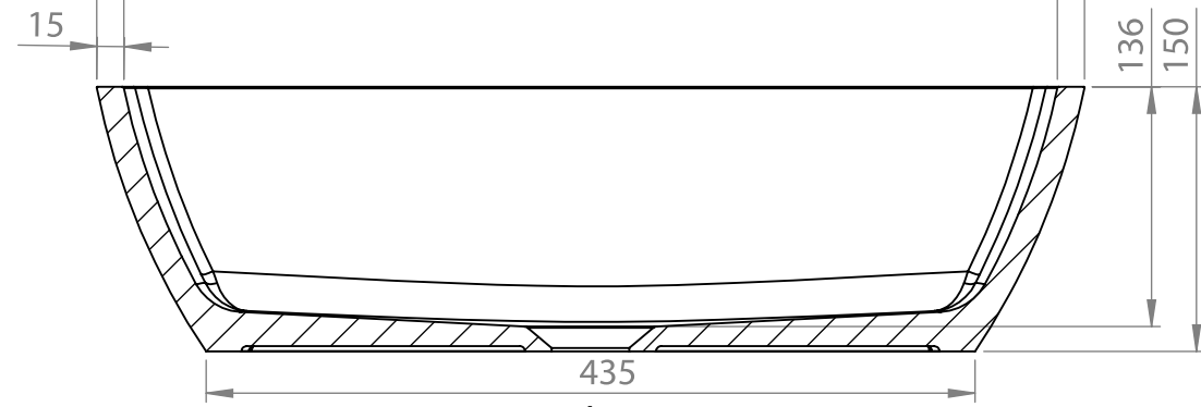
PRZEKRÓJ N-N SKALA 1 : 5
