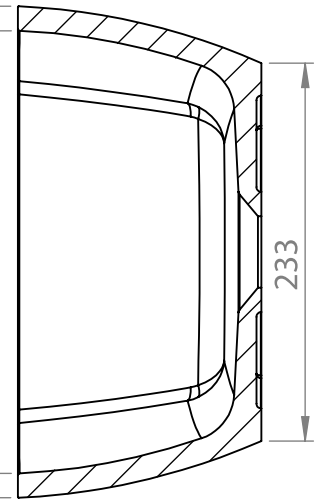
PRZEKRÓJ M-M SKALA 1 : 5
