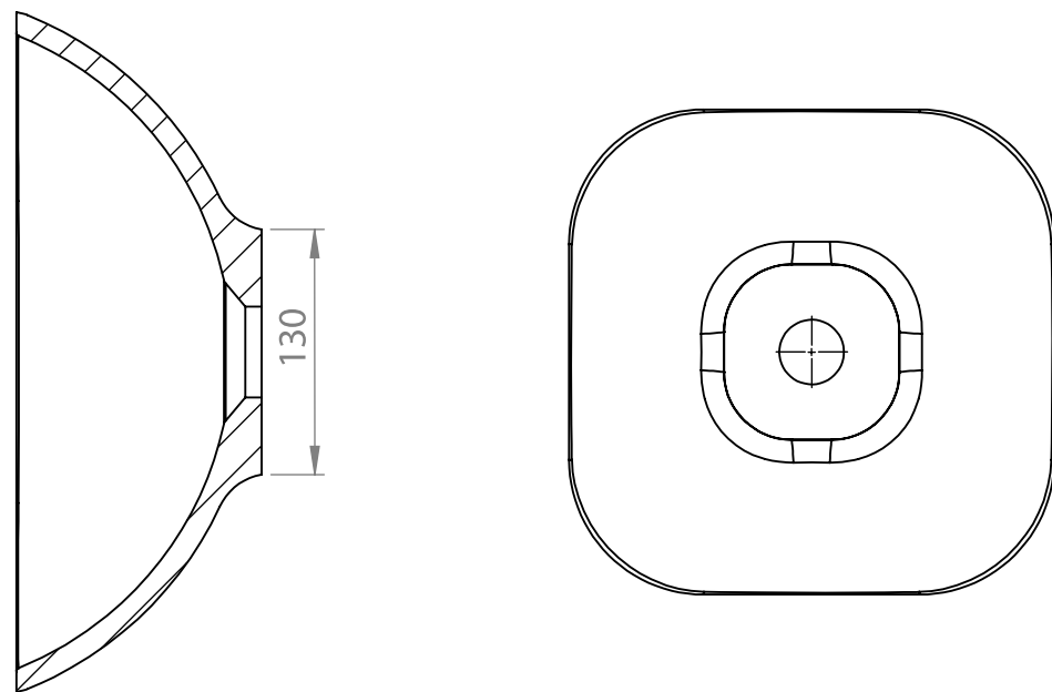
PRZEKRÓJ M-M
