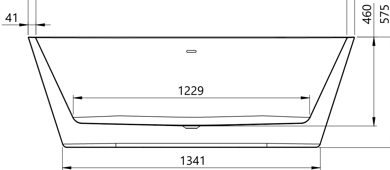
PRZEKRÓJ N-N SKALA 1 : 15
