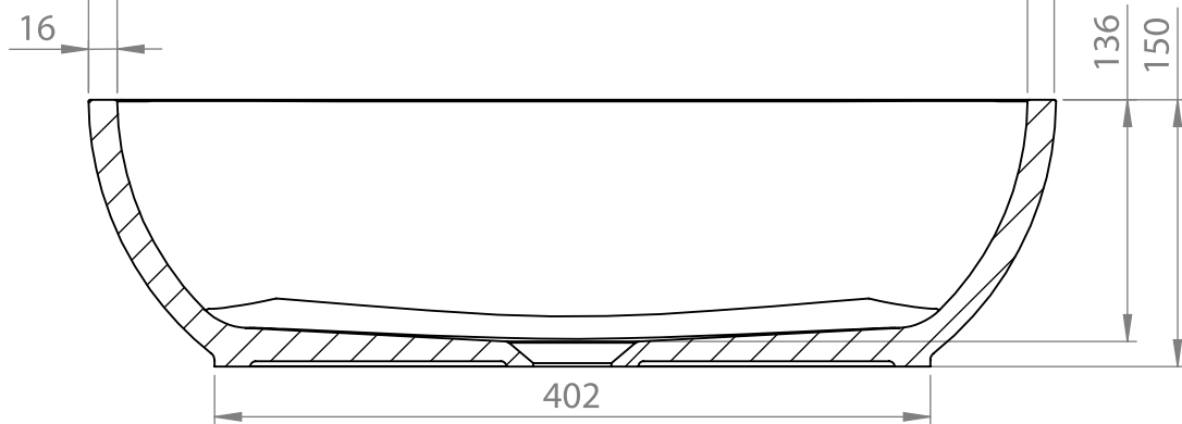
PRZEKRÓJ N-N SKALA 1 : 5
