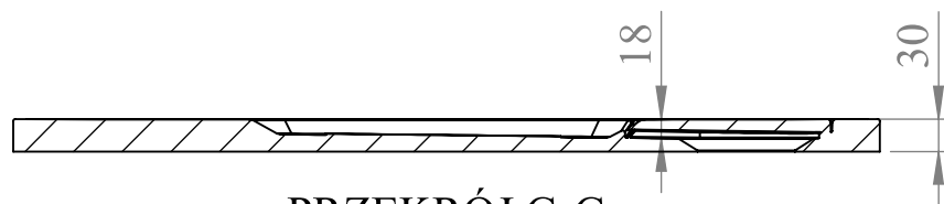
PRZEKRÓJ G-G SKALA 1 : 10
