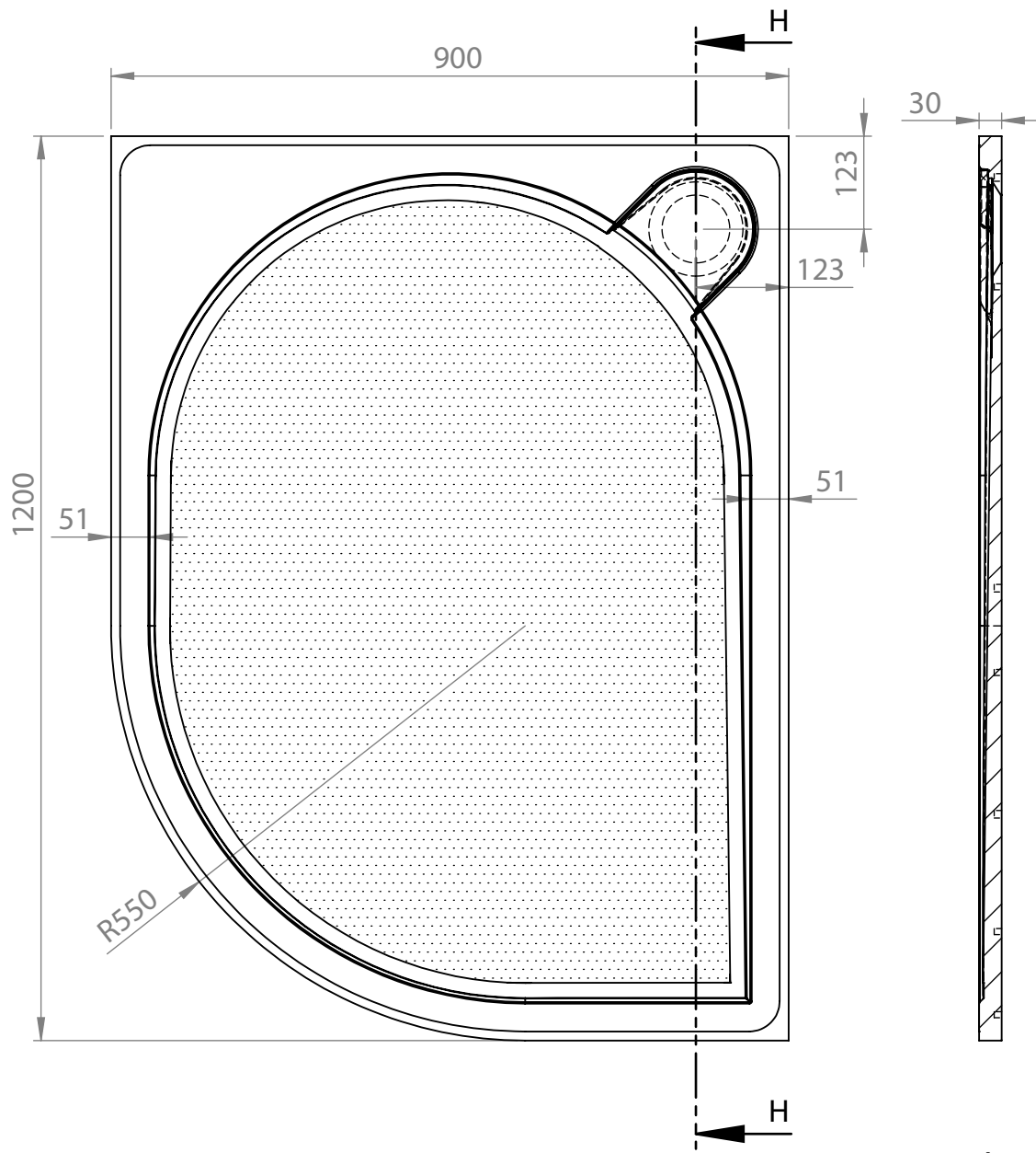
PRZEKRÓJ H-H SKALA 1 : 10
