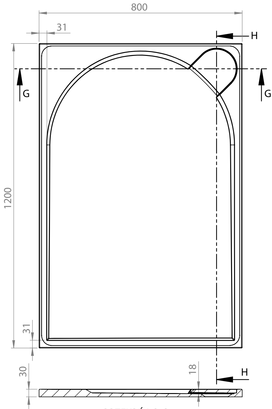
PRZEKRÓJ G-G SKALA 1 : 10
