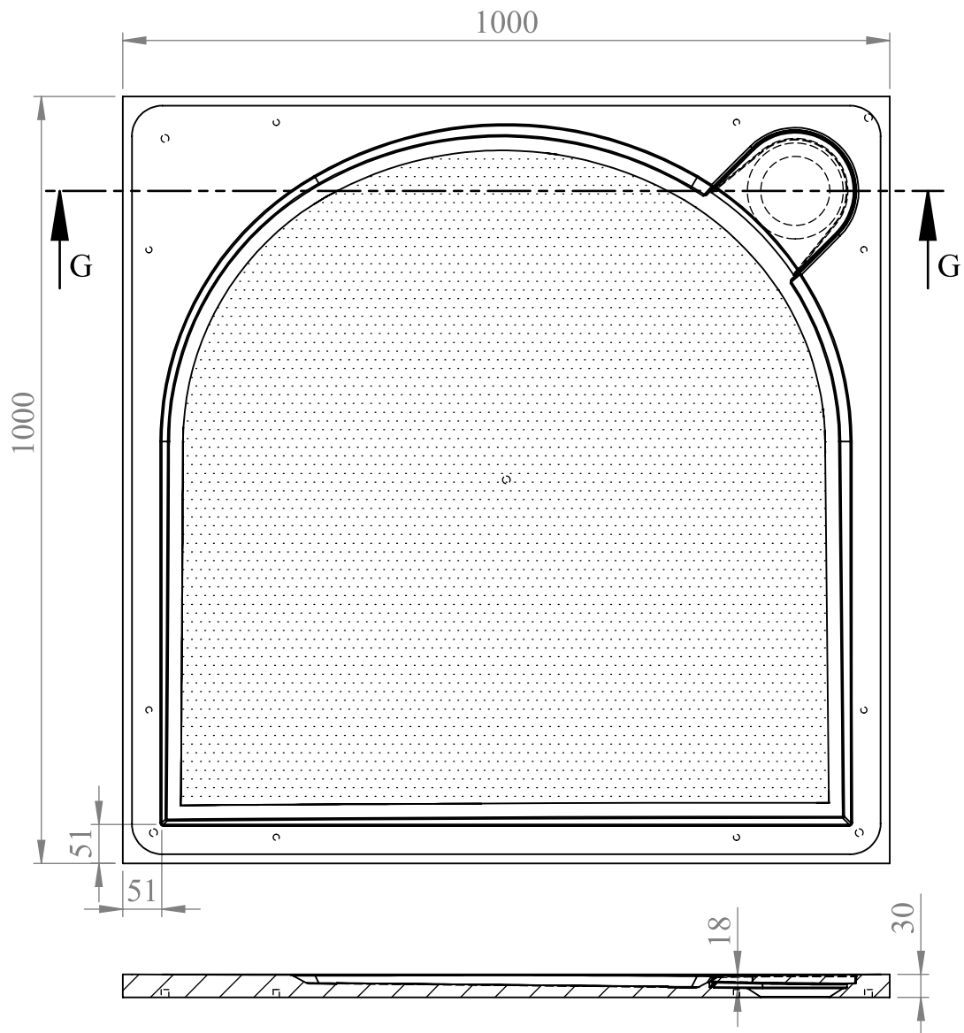
PRZEKRÓJ G-G SKALA 1 : 10
