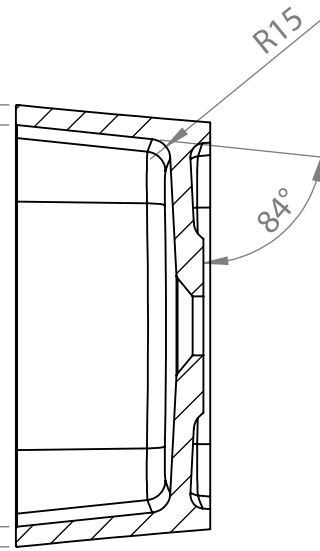
PRZEKRÓJ M-M SKALA 1 : 6
