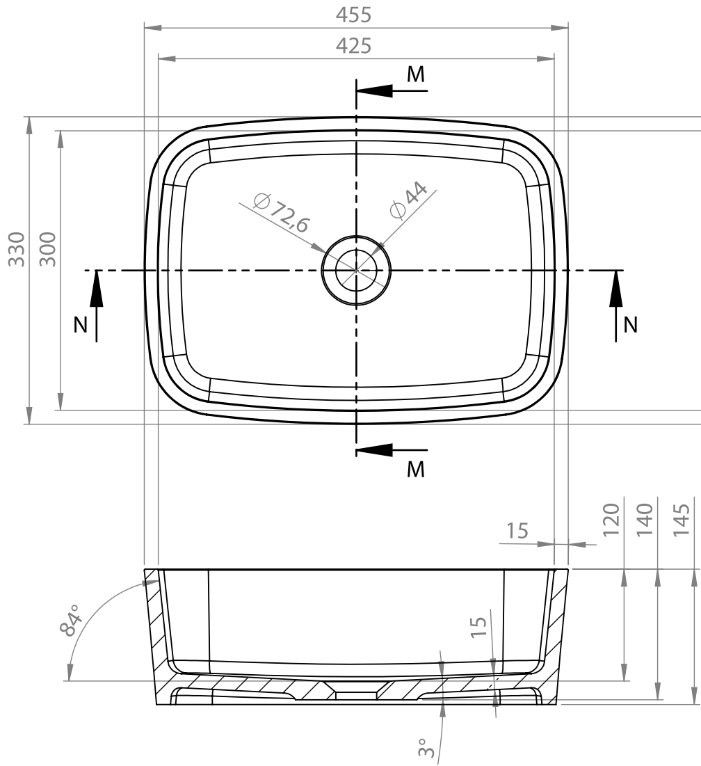
PRZEKRÓJ N-N SKALA 1 : 6
