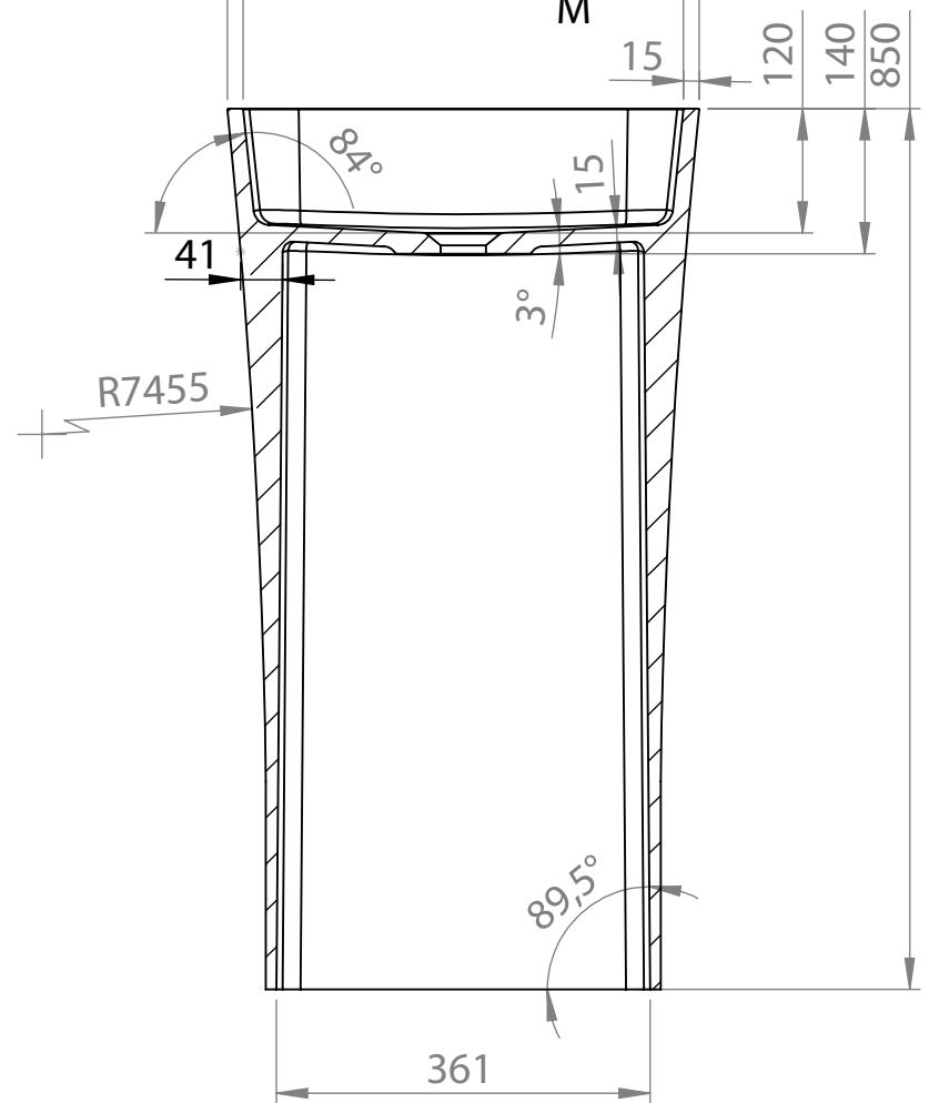
PRZEKRÓJ M-M SKALA 1 : 10
